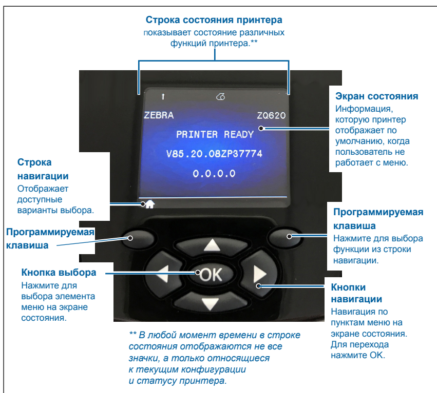
Рис. 16 • ЖК-панель управления
